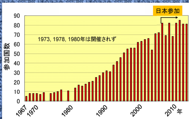
国際物理オリンピック参加国数
