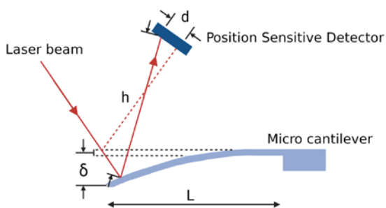
図 1：カンチレバーの変形と位置敏感検出器(Position Sensitive Detector)でのレーザー検出位置の関係を示す模式図
