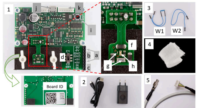
図 1 実験に使用する回路やケーブル等
