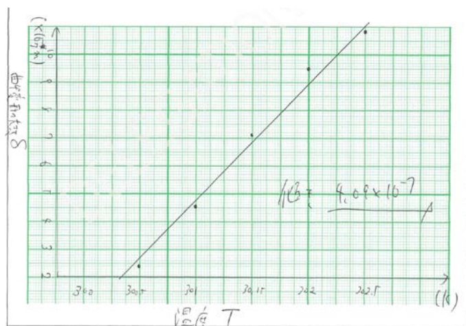
図 2：二重層カンチレバーの変形 \delta と加熱温度 T との関係を示す測定の一例
