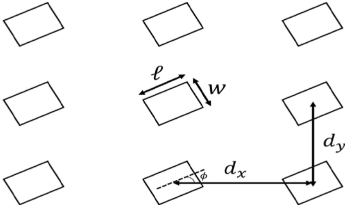
図 3：微小球充填の長方形セルの 3 \times 3 構造の模式図
