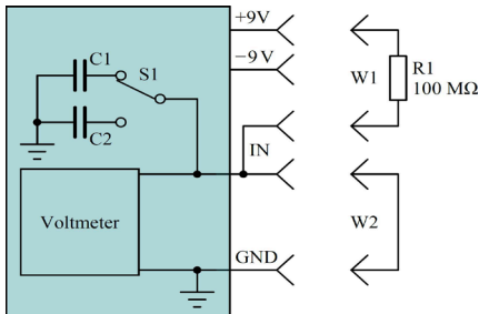
図3 実験問題1の実験回路
