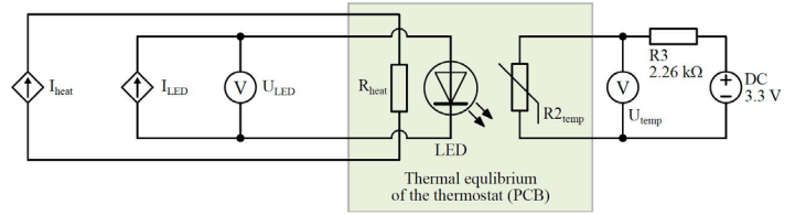
図4 実験問題2の実験回路
