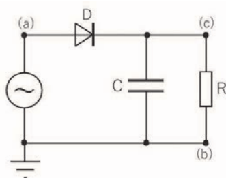
図20 図18にコンデンサを加えた回路
