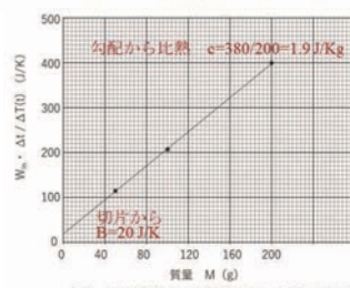
図6 加熱初期における温度変化の勾配の逆数を質量に対してプロットしたグラフ
