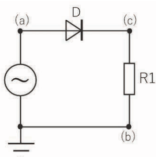
図18 ブラックボックス内に作る回路
