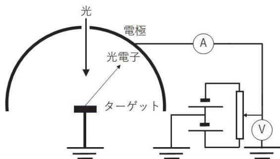
図8 プランク定数測定装置
