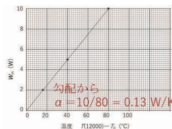
図4 飽和温度に対する電力
