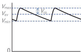
図21 リップル
