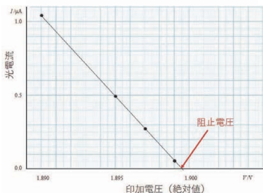
図11 印加電圧に対する光電流の変化 (波長400 nm)
