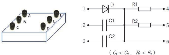
図14 電気ブラックボックス 外観と内部回路
