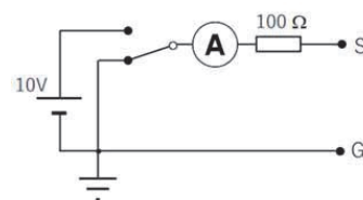
図15 電流計付き 10 V 電源
