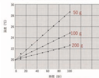
図5 電力10 Wにおける加熱初期の温度変化
