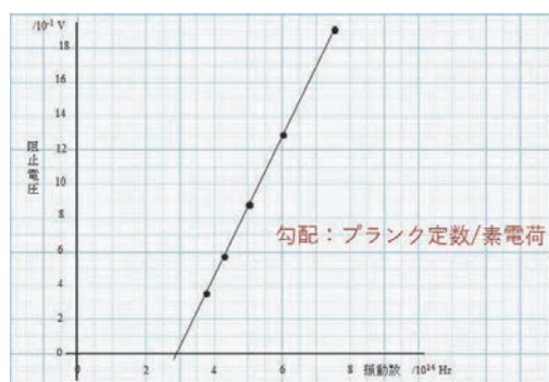
図12 光の振動数に対する阻止電圧の変化
