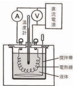
図1 液体の比熱測定装置
