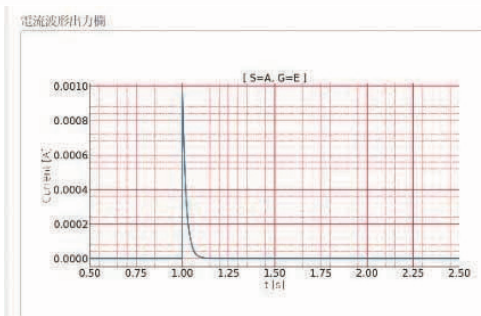
図17 図16の入力に対する応答
